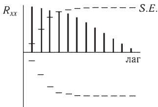
Рис. 1. Графік R_{xx} , характерний для АРКС-процесу
