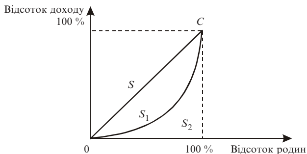
Рис. 10.6. Коefіцієнт Джині
